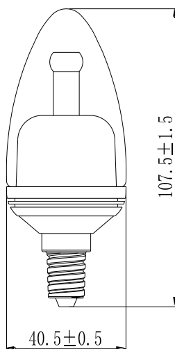
Fig 1. E14 Base
